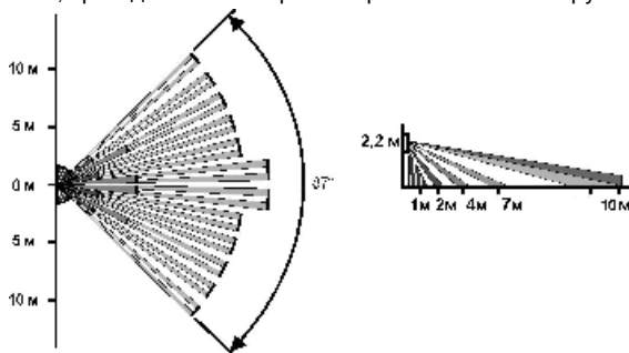
Рис.5 Диаграмма зоны обнаружения
